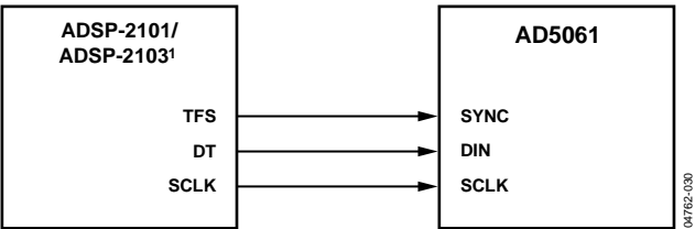
Figure 31. AD5061-to-ADSP-2101/ADSP-2103 Interface
