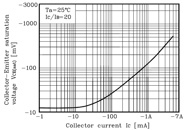
Fig. 4 V_{CE(sat)} - I_c
