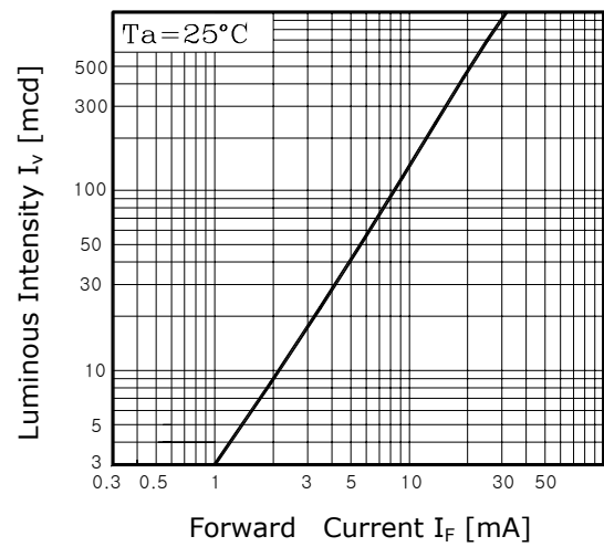
Fig. 2 I_V - I_F
