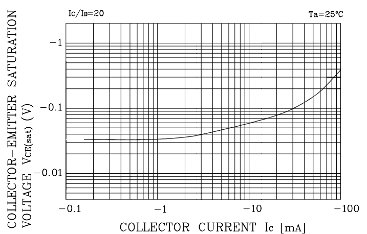
Fig. 2 V_{CE(SAT)} - I_C
