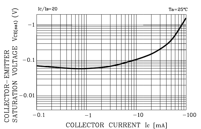
Fig. 2 V_{CE(SAT)} - I_C
