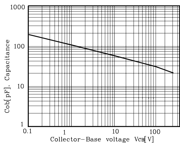
Fig. 6 Capacitance
