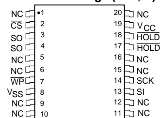
TSSOP Package (U20, Y)**
