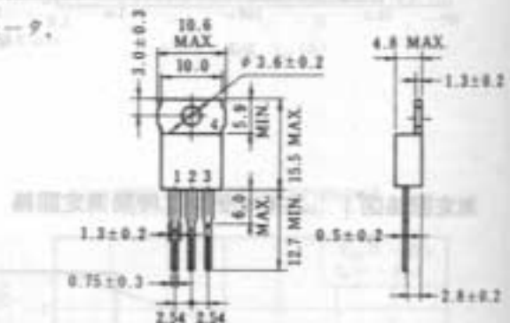
電極接続
