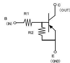
等価回路
