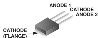
JEDEC TO-251AA
