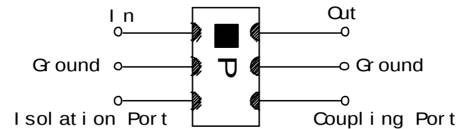
1.92/1.98GHz Band Chip Multilayer Coupler“FSLC-S190E-W”
