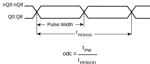
odc & t_{PERIOD}
