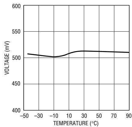
Charge Enable Threshold (V CC – BAT)
