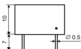
Рис.2 Корпус пластмассовый
