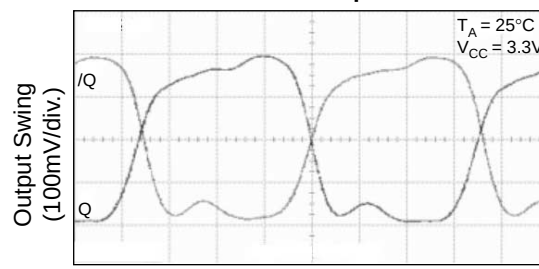
2GHz Output
