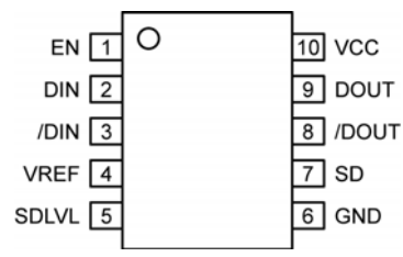
10-Pin EPAD-MSOP (K10-2)
