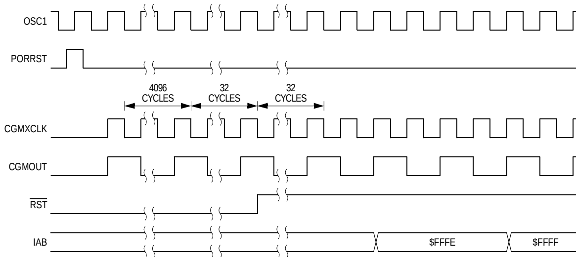
Figure 9-7. POR Recovery
