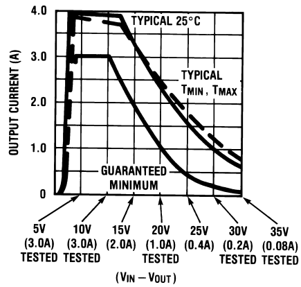
LM333 Guaranteed Output Current
