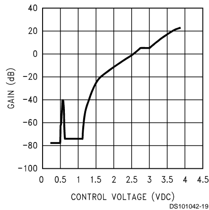
Attenuation Level vs DC-Vol Amplitude
