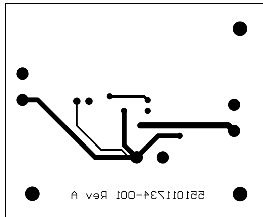
Bottom Layer
