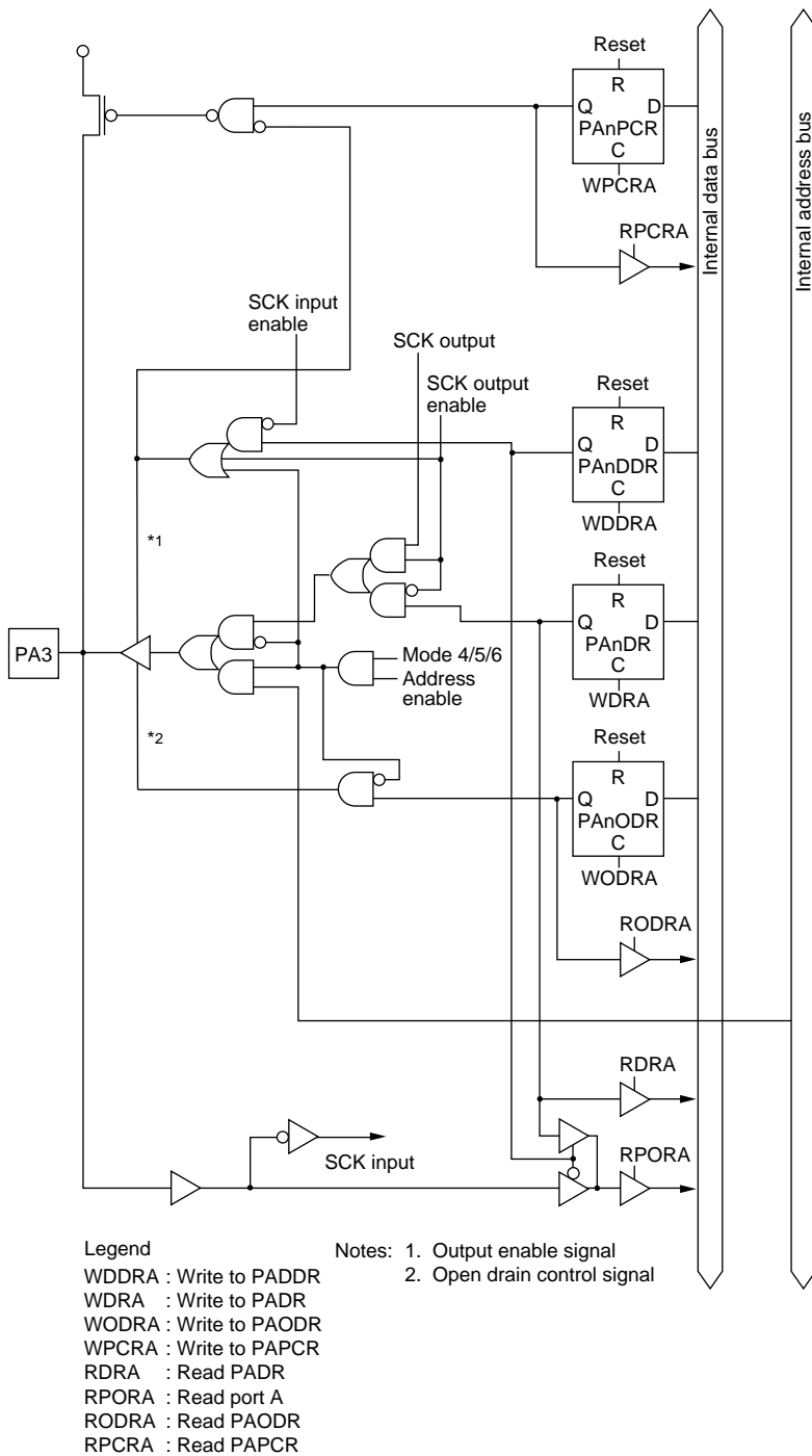
Figure C-9 (d) Port A Block Diagram (Pin PA3)
