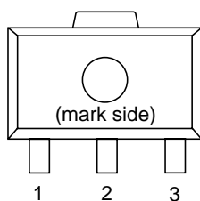
• SOT-89
