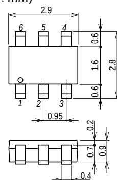
外形図 2146A (unit : mm)
