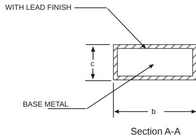
16 PIN SSOP
