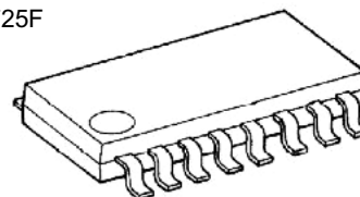
SSOP16-P-225-1.00
