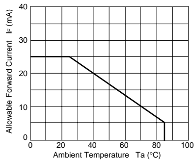
If – Ta
