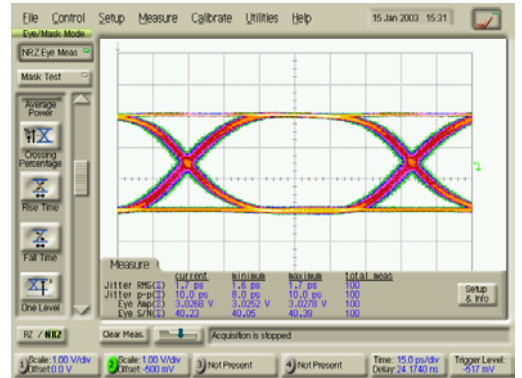
Vo=3V
