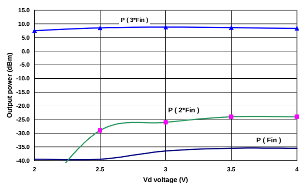
Pout versus Vd @ Pin=14dBm &amp; Fin=12GHz
